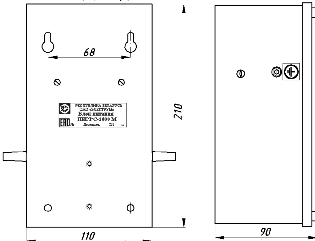
Блок питания (вид снизу)
