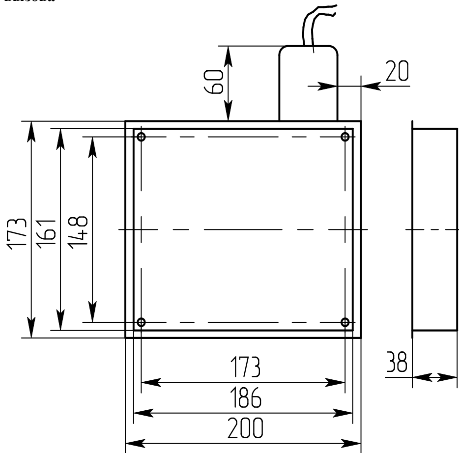
Блок питания (вид снизу)
